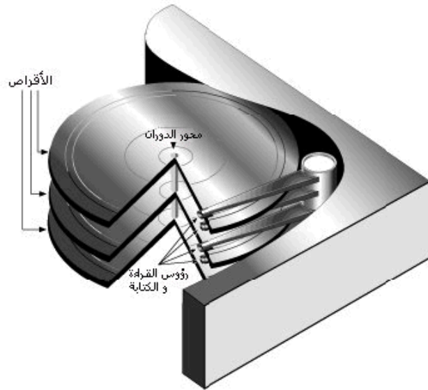
الشكل 1: المكونات الأساسية للقرص الصلب
