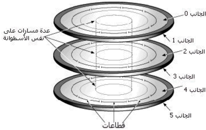
الشكل 2: الهيئة الفيزيائية لقرص صلب نموذجي
